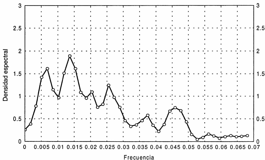
Figura 3. Densidad espectral de la serie de precipitación mensual media del período 1951-1999 en función de la frecuencia (ciclos/mes).
