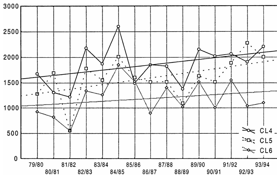
Figura 10.b). Rendimientos (kg ha -1 ) de trigo para los clusters Cl4, Cl5 y Cl6.
