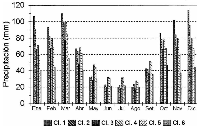
Figura 7. Onda anual de la precipitación mensual (mm) para cada uno de los 6 clusters de la RESAP.
