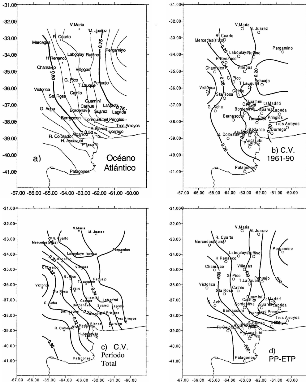
Figura 1. a), b), c) y d). La Región Semiárida Pampeana (RESAP), a) localidades e Índice de Aridez, b) Coeficiente de Variación (C.V.) de la precipitación para el período 1961-1990, c) C.V. para el período total y d) déficit hídrico (mm).
