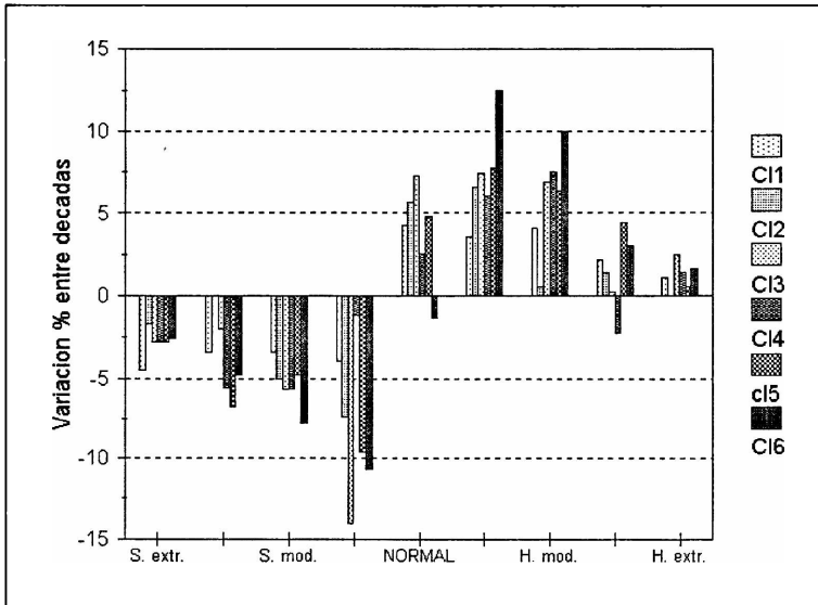
Figura 8. Variación porcentual de las condiciones de déficits o excesos hídricos por categorías del IPE3 (ver texto) y por clusters, entre los períodos 1911-40 y 1970-99.
