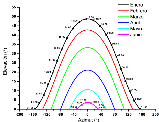
Figura 2. Trayectoria solar en la Base Marambio para diferentes meses del año.
