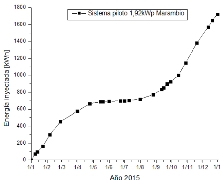
Figura 6. Perfil de generación de energía eléctrica a lo largo del año 2015. En la integral anual el valor de energía inyectada fue de 1720kWh.
