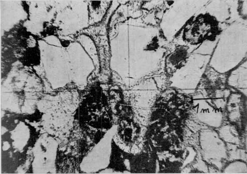
Fig. 6. — Cemento de analcima (zonas gris claras) que une elastos de plagioclasa, cuarzo y líticos. Contra los elastos se distingue un delgado reborde de la matriz tobácea que no ha sido reemplazada por la zeolita. Luz paralela.
