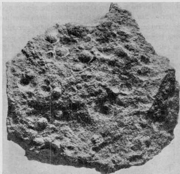
Fig. 1. — Toba fina con cuerpos esferoidales (cuasi-oolitas) de analcima que cementa trizas vítreas. Aproximadamente tamaño natural
