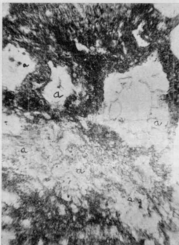
Fig. 3. — Analcima que rellena parcialmente cavidades y forma franjas de reemplazo en la base piroclástica. Luz paralela
