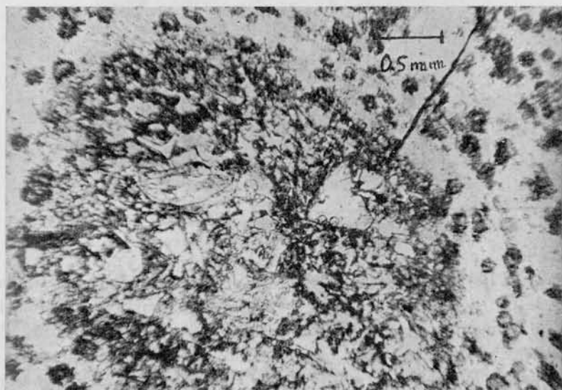
Fig. 2. — Una cuasi-oolita en la base tobácea. Se observan las trizas de vidrio y la presencia de cuerpos pequeños de analcima en la matriz (gris oscuro). Luz paralela
