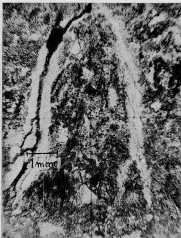
Fig. 4. — Dos venillas convergentes de analcima. La zeolita se encuentra también entre las venas, pero no se distingue en la fotografía. Luz paralela
