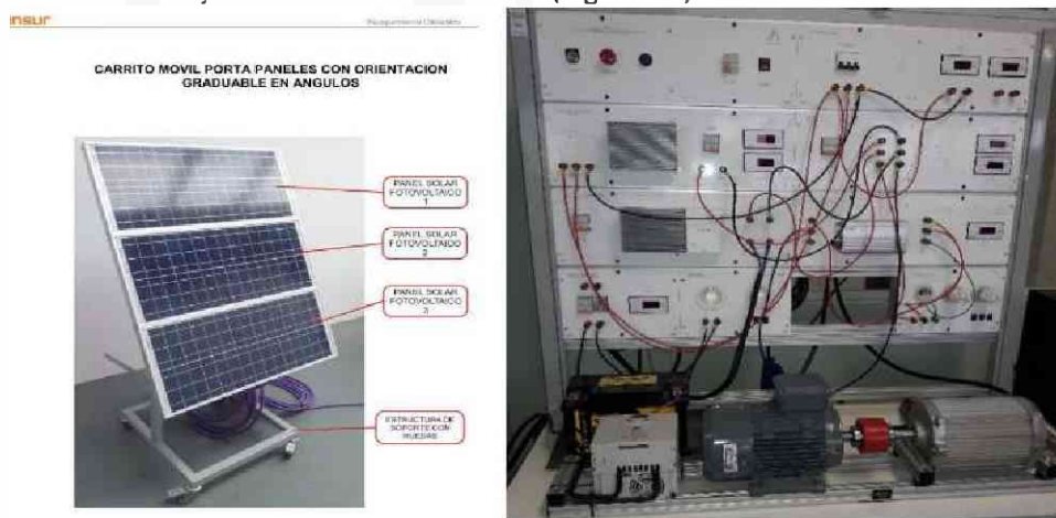
Figura 9: Simulador de Energía Solar Fotovoltaica (izq) y Simulador eólico con variador, motor y generador
