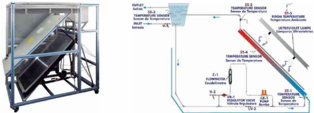
Figura 1: Diagrama del equipo MiniEESTC (derecha) y foto del mismo (izquierda)
