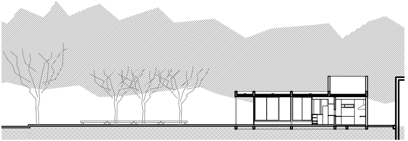
CORTE TRANSVERSAL PLAZA Y EDIFICIO
