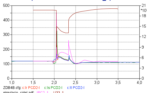
ZDB4B.cfg: c:Ir PCD2-I c:Is PCD2-I c:It PCD2-I simulacio_cidel.adf: IPC2_1 U33_1 Figura 9. Corriente eficaz de un alimentador de 33kV Barra I. Valores registrados (evento 42) de las tres fases y simulada (secuencia directa PCD2_1). Tensión simulada barra I en 33 kV, U33_1
