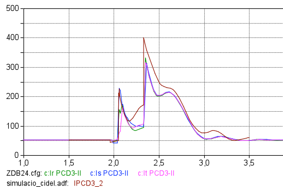
ZDB24.cfg: c:Ir PCD3-II c:Is PCD3-II c:It PCD3-II simulacio_cidel.adf: IPCD3_2 Figura 8. Corriente eficaz de un alimentador de 33kV Barra II. Valores registrados (evento 42) de las tres fases y simulada (secuencia directa PCD3_2)
