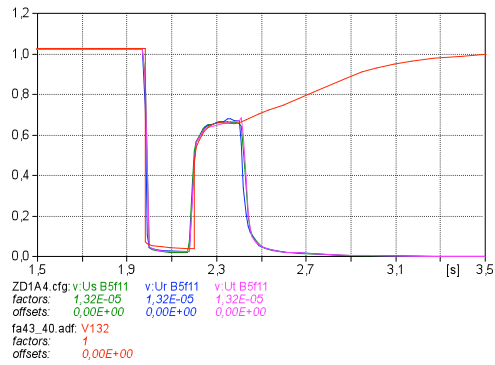
Figura 3. Tensión eficaz de 132 kV de las tres fases (evento 39) registrada y la secuencia directa simulada (V132).
