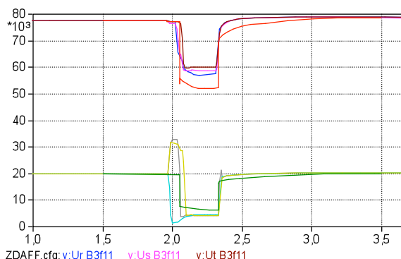
ZDAFF.cfg: v:Ur B3f11 v:Us B3f11 v:Ut B3f11 ZDB24.cfg: v:Ur Barra III v:Us Barra III v:Ut Barra III simulacio_cidel.adf: U132 U33_2 Figura 7. Tensión de 132 kV y 33 kV de las tres fases (evento 42) registrada y tensiones de secuencia directa simuladas (U132, U33_2).
