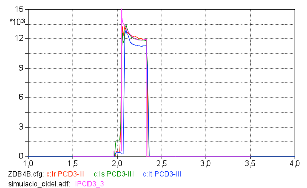
Figura 6. Corriente de falla del alimentador de barra III de 33 kV (evento 42), las tres fases registradas y corriente de secuencia directa simulada (IPCD3_3).
