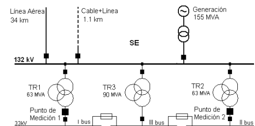
Figura 1: Esquema general de la S.E. y ubicación de los puntos de medición
