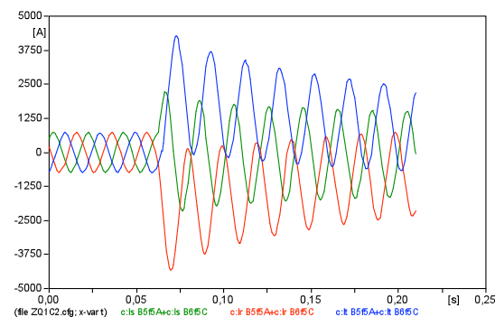
Figura 5. Registro de corriente instantánea entregada por el Generador en 132 kV de las tres fases correspondiente al evento 39.
