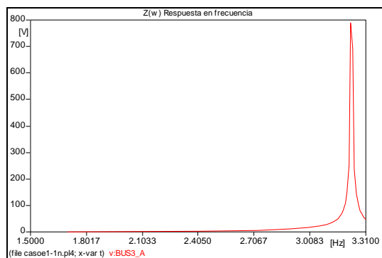
Figura 2. Respuesta en frecuencia en la barra N°3, sin filtros
