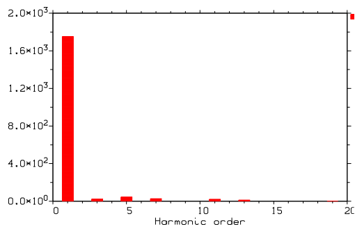
Figura 7. Contenido armónico - Caso Sin Filtros.
