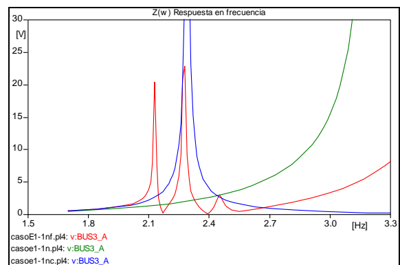
Figura 5. Respuesta en frecuencia en la barra N°3. Comparación de los casos analizados.
