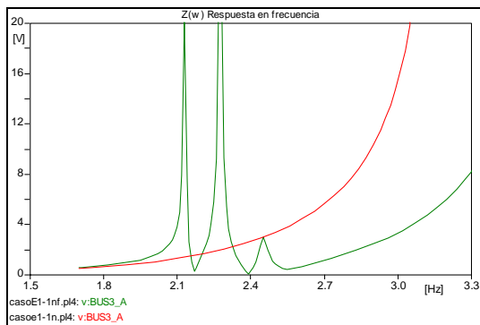
Figura 3. Respuesta en frecuencia con todos los filtros, y comparación con el caso base.
