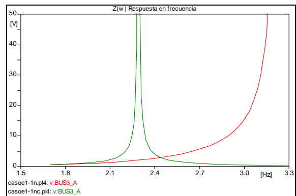
Figura 4. Caso con compensación capacitiva, comparado con el caso base.
