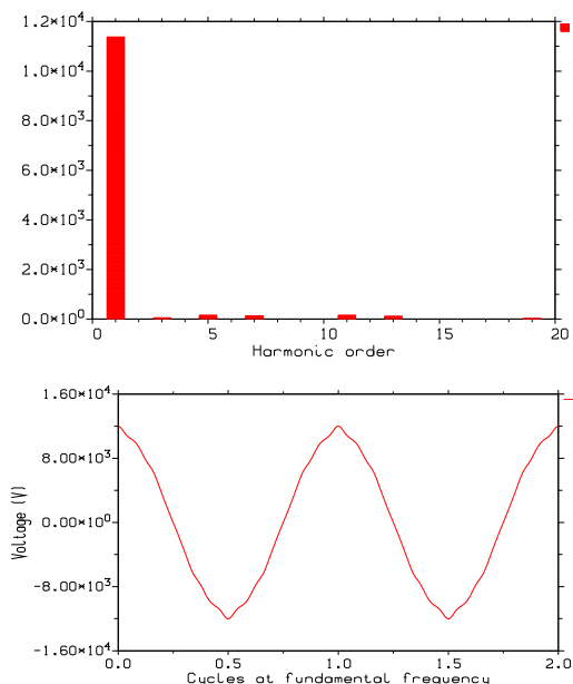
Figura 6 a) Contenido armónico y b) forma de onda de la tensión en Barra N°3 - Caso Sin Filtros.
