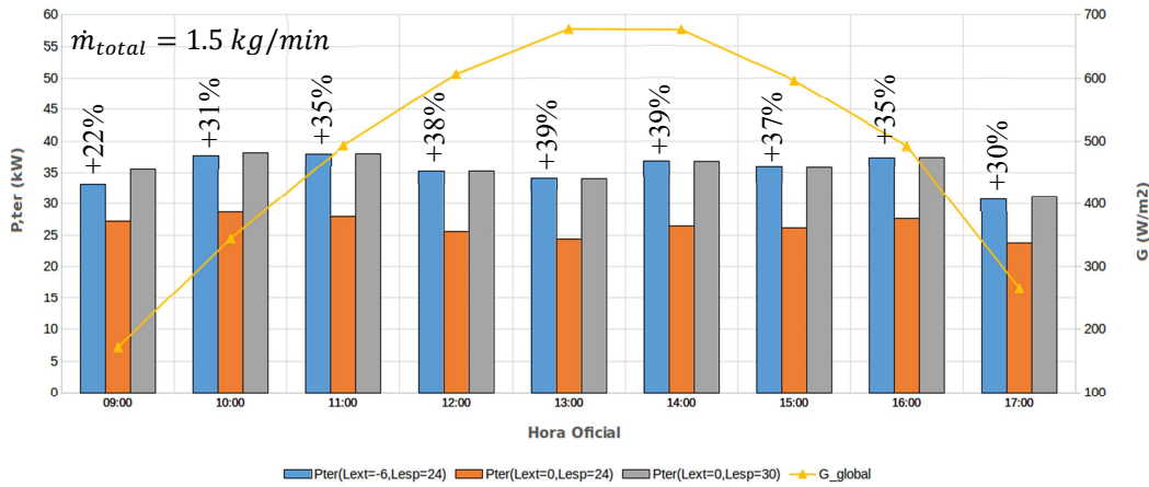
Figura 6: P_{ter}(kW) generada por el LFC para el 21 de Junio, tres casos de comparación.
