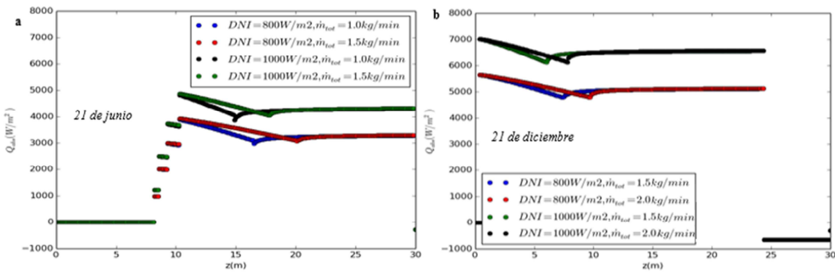
Figura 5: Q''_{abs} vs z para 12:00 hora solar y DNI = 800 \text{ W/m}^2, 1000 \text{ W/m}^2 : a) 21 de Junio ( \dot{m}_{total} = 1.0 \text{ kg/min}, 1.5 \text{ kg/min} ) y b) 21 de Diciembre ( \dot{m}_{total} = 1.5 \text{ kg/min}, 2.0 \text{ kg/min} ).
