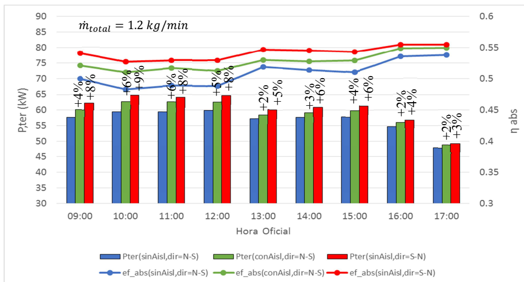
Figura 9: P_{ter}(kW) generada por el LFC y \eta_{abs} , para el 21 de Diciembre (tres casos de comparación, \dot{m}_{total} = 1.2 \text{ kg/min} ).
