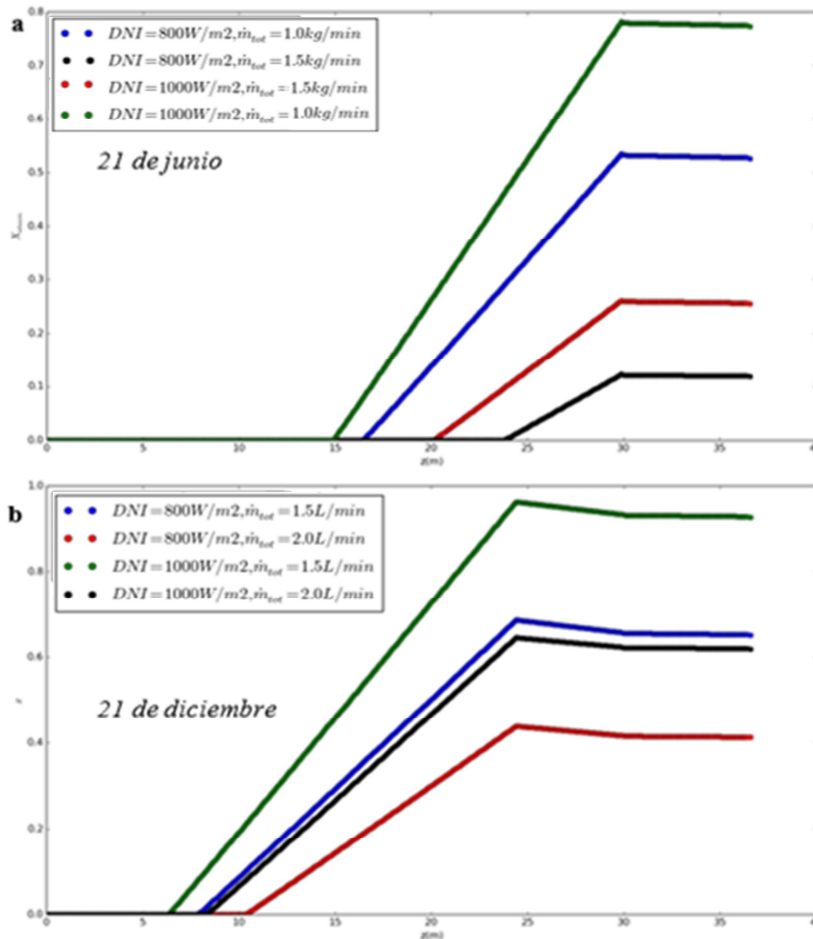
Figura 4: Evolución de la fracción de vapor ( x ) con z para las 12:00 hora solar y DNI = 800 W/m^2, 1000 W/m^2 : a) 21 de Junio ( \dot{m}_{total} = 1.0 kg/min, 1.5 kg/min ) y b) 21 de Diciembre ( \dot{m}_{total} = 1.5 kg/min, 2.0 kg/min ).
