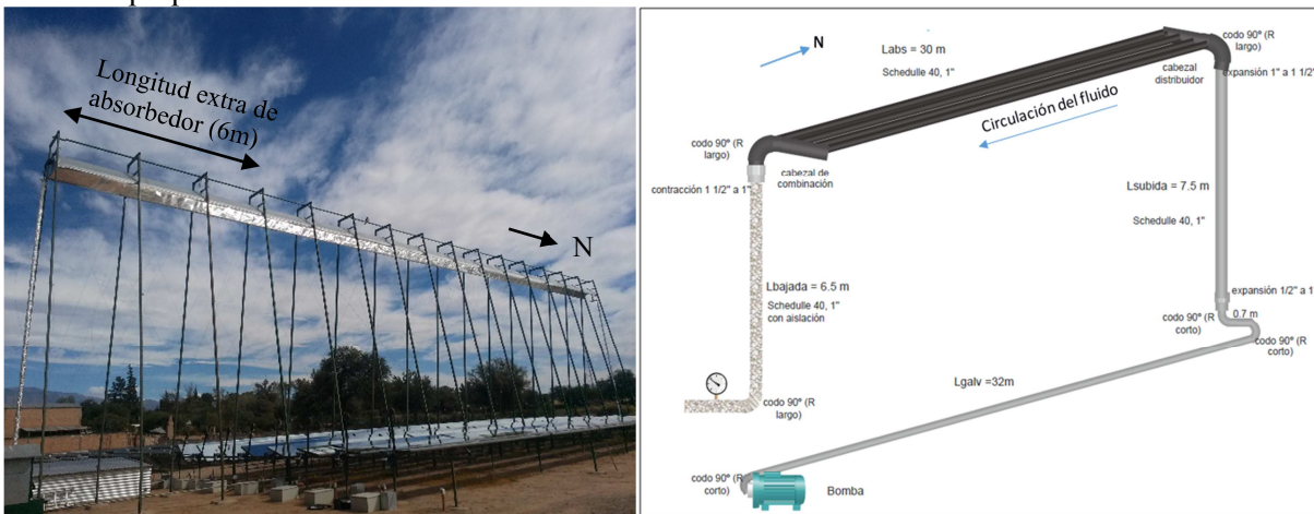
Figura 1: a) Concentrador Fresnel Lineal de 173 \text{ m}^2 instalado en San Carlos, Salta. En b) circuito hidráulico simulado.
