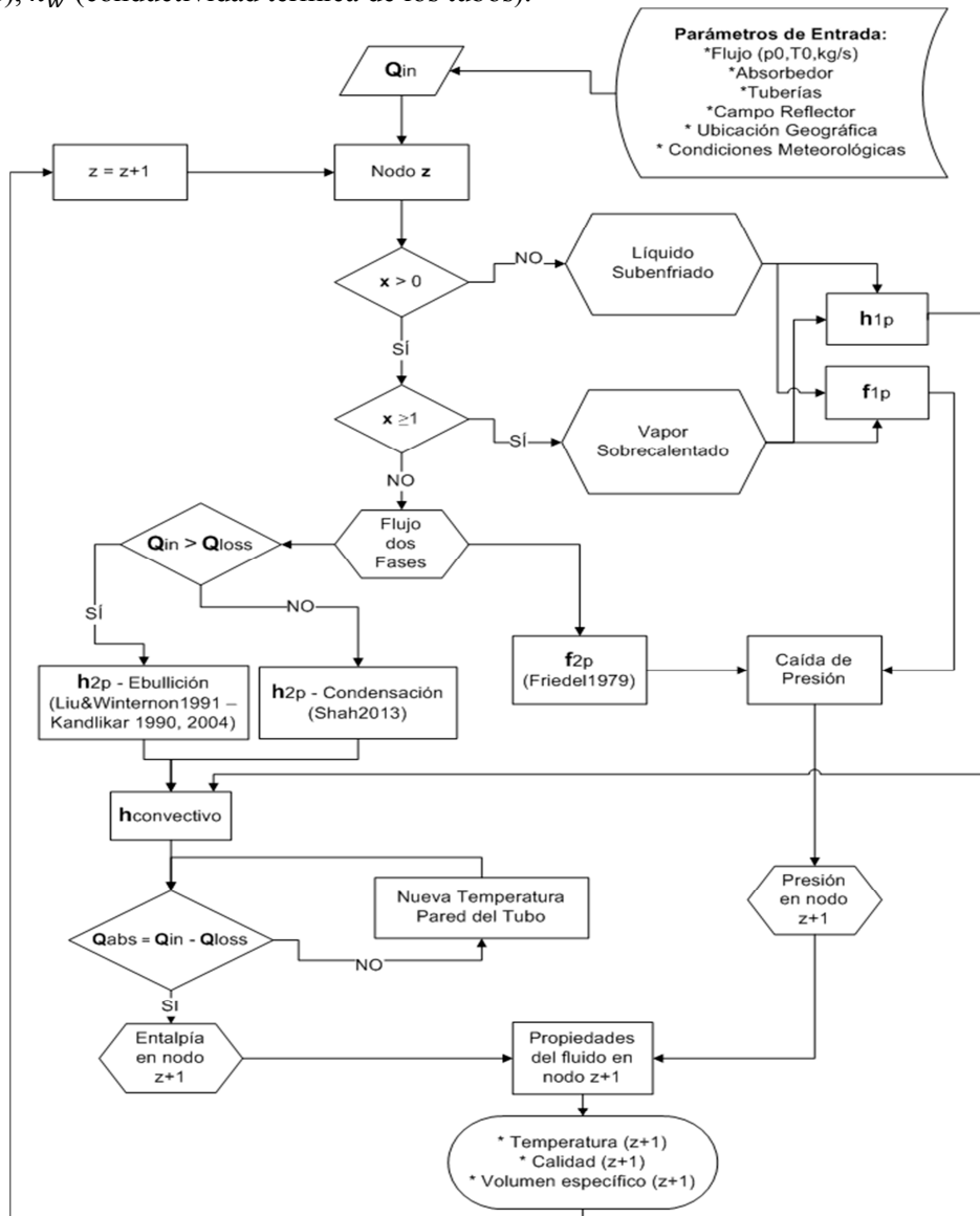
Figura 2: Algoritmo y procedimiento de cálculo empleado por el modelo.
