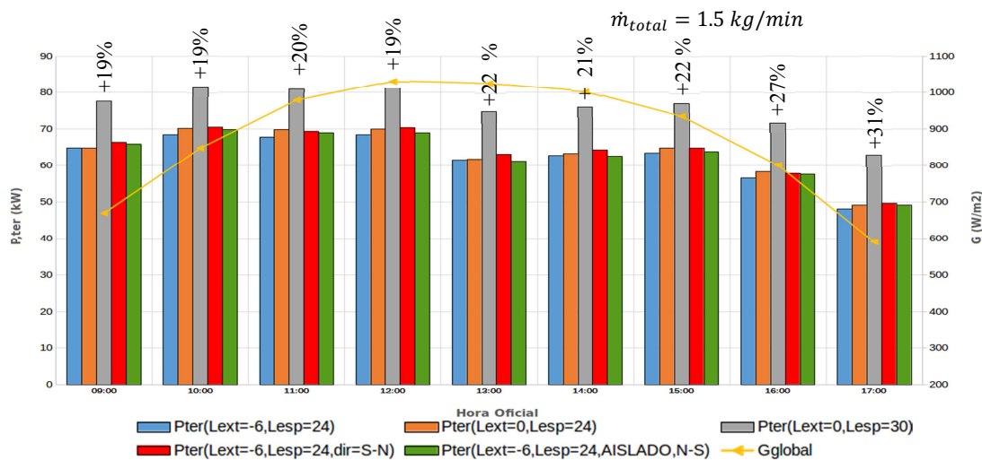
Figura 8: Eficiencia térmica global ( \eta_{global} ), para el 21 de Diciembre (cinco casos de comparación, \dot{m}_{total} = 1.5 kg/min).
