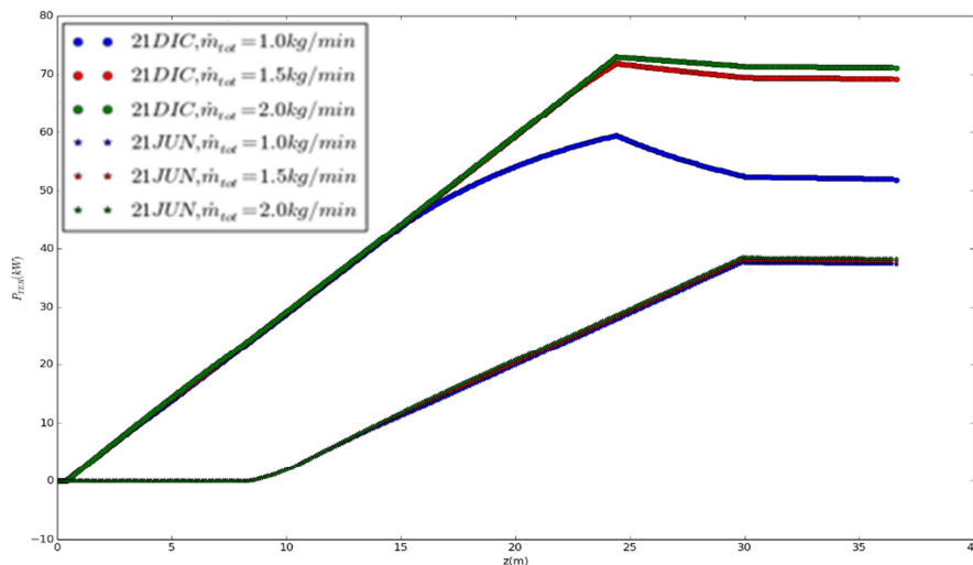
Figura 3: P_{ter} (kW) vs z para el 21/06 y 21/12, para diferentes valores \dot{m}_{total} . DNI = 1000 \text{ W/m}^2 , 12:00 hora solar.
