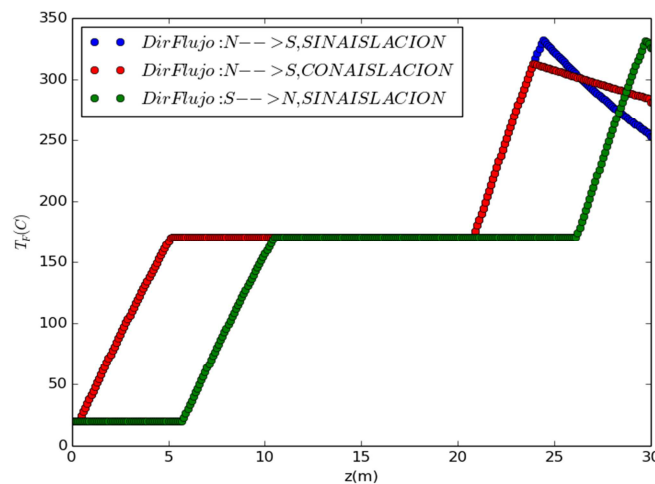
Figura 10: Perfil de temperatura T_f para el 21/12 al medio día solar ( \dot{m}_{total} = 1.2 kg/min), tres casos de funcionamiento: caso actual (azul), longitud extra de absorbedor aislada térmicamente (roja) y cambio en dirección de flujo sin aislación (verde).
