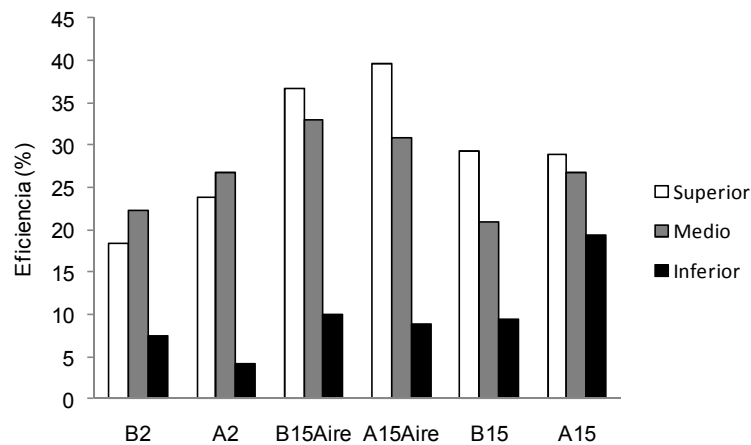
Figura 9. Eficiencia sobre el haz de las hojas para los diferentes tratamientos en los distintos estratos del cultivo. A: mayor tasa de aplicación; B: menor tasa de aplicación; 2: CH8002; 15: CH80015; 15Aire: TVI80015.
